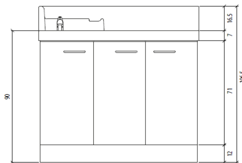
ELEVATION LAVABO GAUCHE
