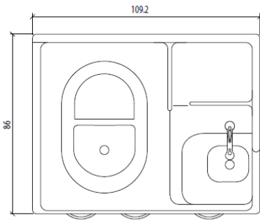
PLAN LAVABO A DROITE
