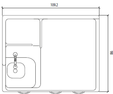
PLAN LAVABO GAUCHE
