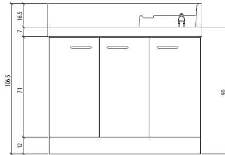
ELEVATION LAVABO A DROITE
